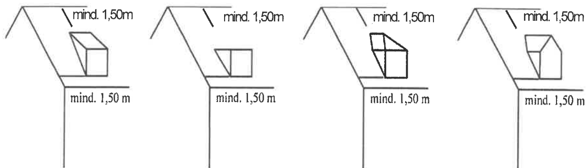
SCHLEPPGAUBE
